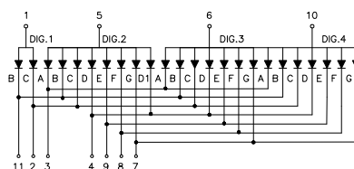
FYQ-3641Hx
